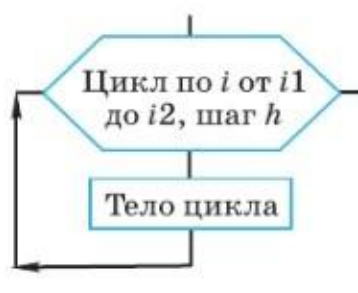
Рис. 3.14. Цикл с переменной
