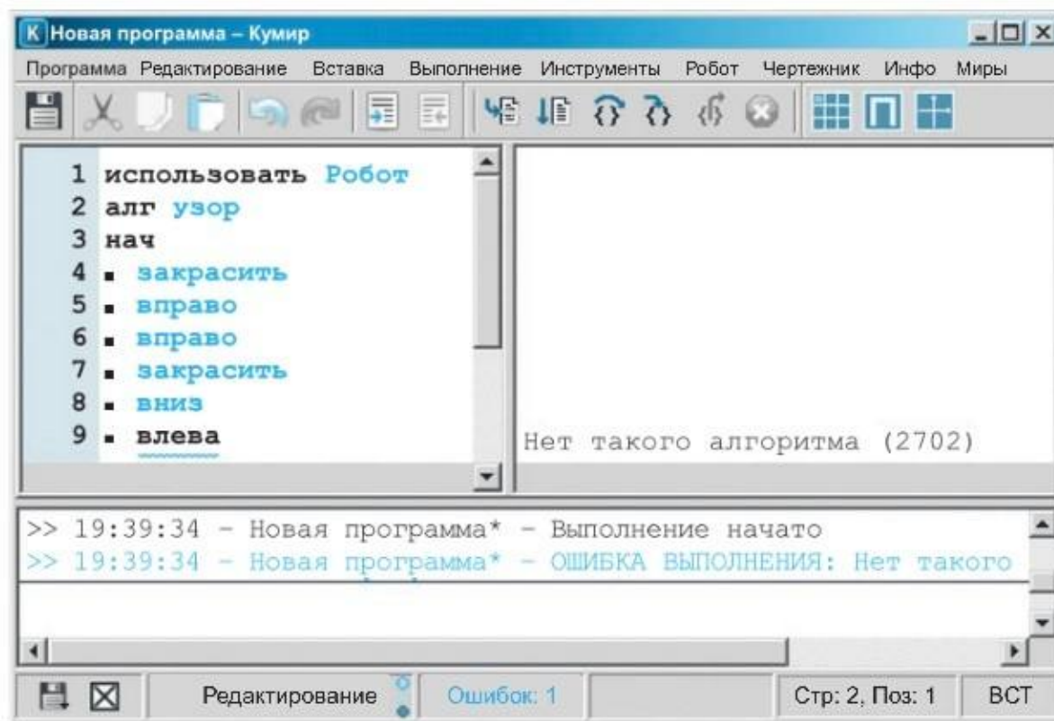
Рис. 3.9. Синтаксическая ошибка в алгоритме
