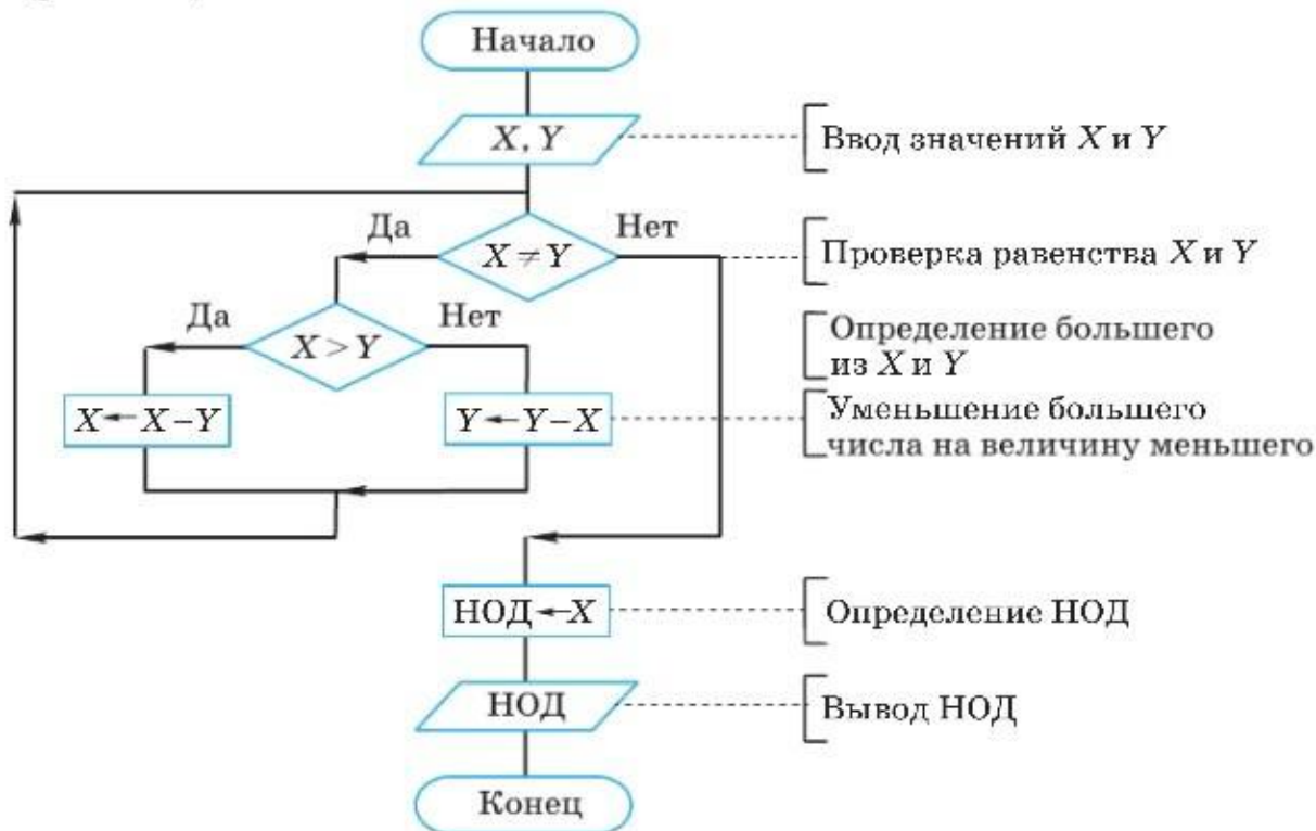
Рис. 3.3. Запись алгоритма Евклида с помощью блок-схемы
